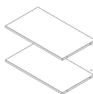
2 Estantes + Trasera M 700 x 400 x 380 mm
