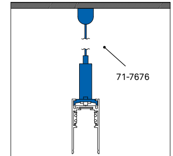
Installation / Instalación
