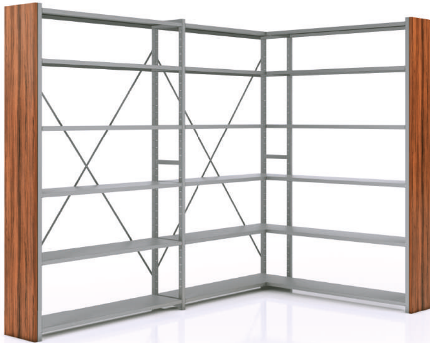
En este caso la estantería está configurada con unas pletinas de uniones para poder hacer módulos en esquina
